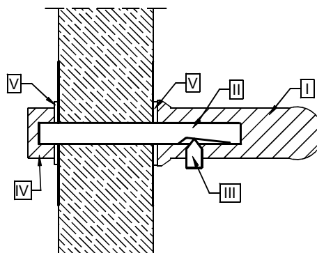
Schemat montażu elementów Przekrój A-A
